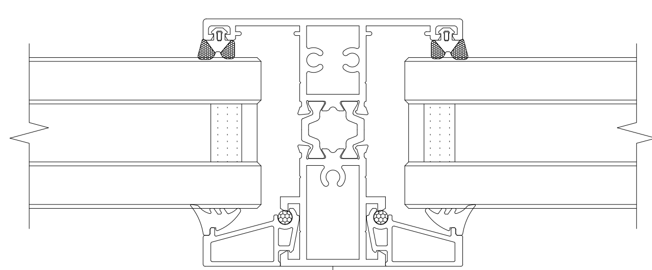
固玻中柱 ZS-ZZ-YZ036
